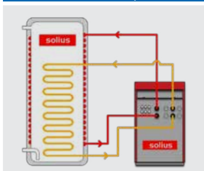
Acumulador sanitário com recuperador
