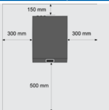
Dimensões mínimas de instalação
