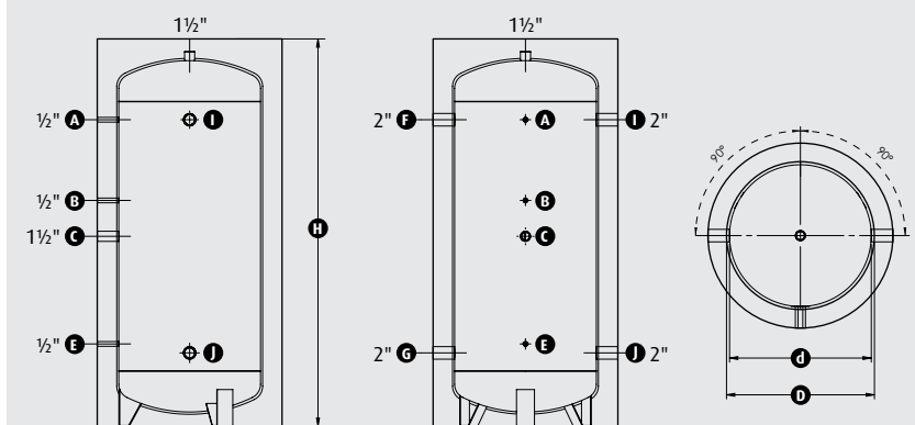
Dimensões 800L a 2000L (mm)
